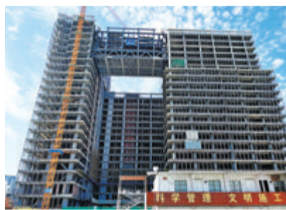
960吨的钢构连廊被安全提升至安装位置。(永富建工 供图)
