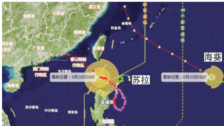
上午8时台风“苏拉”和“海葵”的中心位置。中央气象台发布
